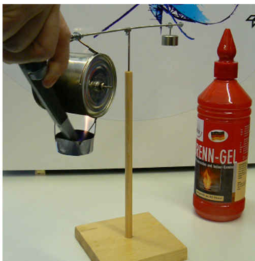
Abb. 6: Entzünden der Brennpaste zum Start des Triebwerks
